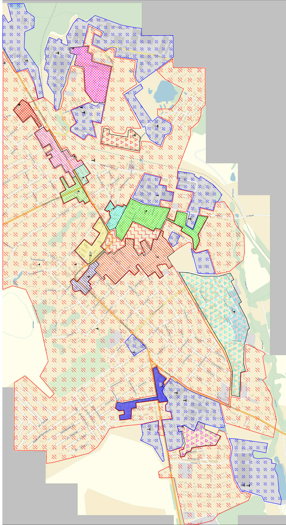
Рис. 1. Зоны действия источников тепловой энергии г. Малоярославцы
